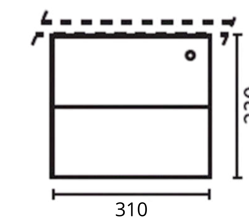
Gaveteiro fixo (2 gavetas) Profundidade: 400mm
