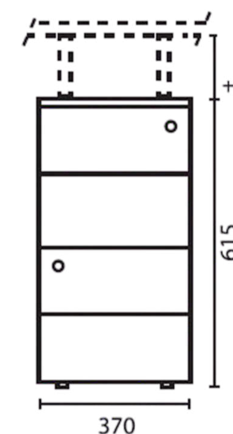
Gaveteiro pedestal (Compartilhado - 4 gavetas e 2 fechaduras)
