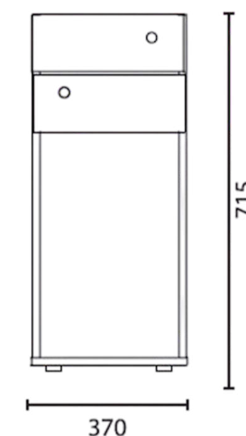
Gaveteiro pedestal (2 gavetas - Nicho para CPU)
