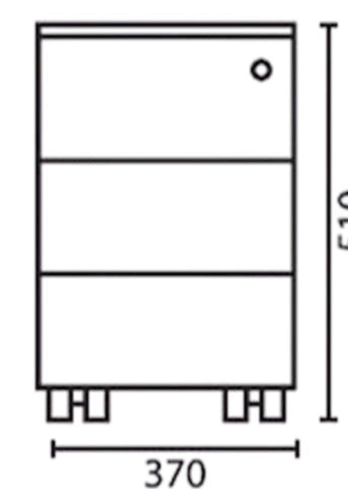
Gaveteiro volante (3 gaveta) Profundidade: 400mm
