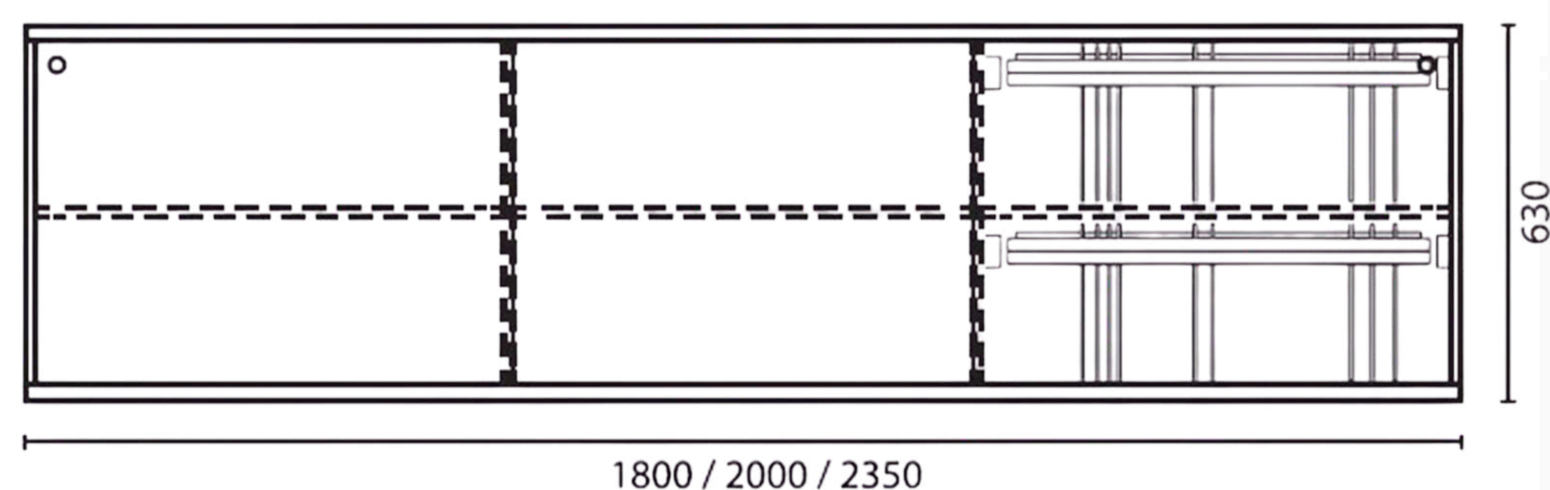
Credenza (3 vãos) 2 portas
